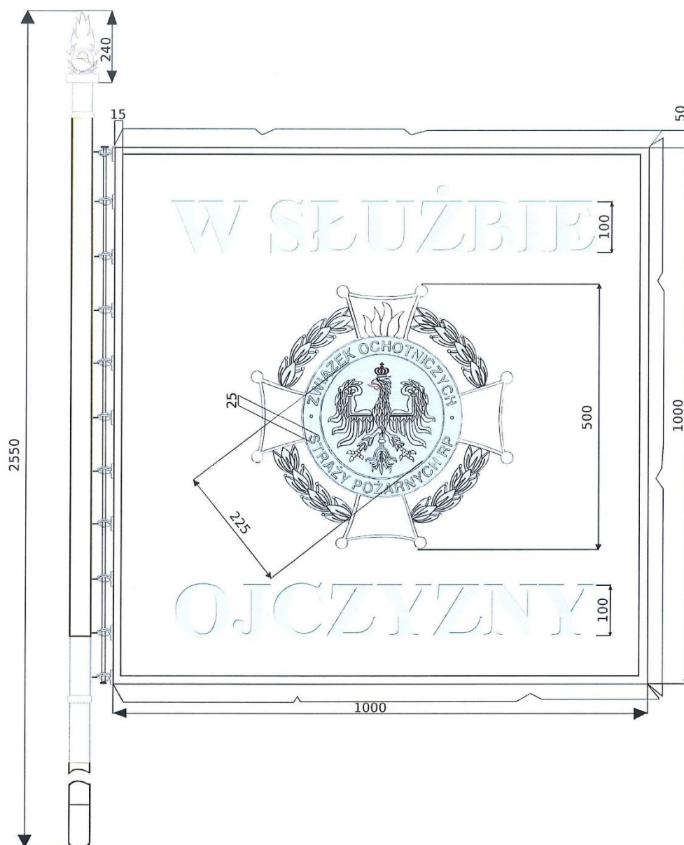
Strona główna (awers) płata sztandaru
